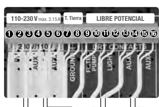
AUX 1 3 y 4 Base (bomba)* o Ultravioleta (según modelo) AUX 2 5 y 6 redoX / Cloro Libre ppm's (bomba) AUX 3 13 y 14 AUX 4 Control calefacción 15 y 16
