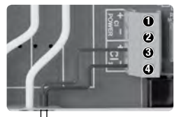
Sonda Cloro Libre 3 rojo 4 negro
